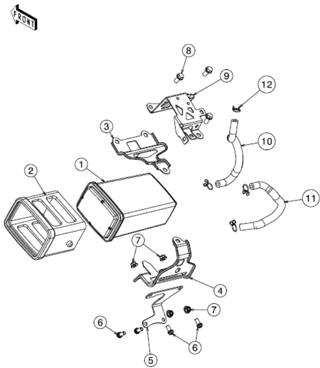
19 Canister
