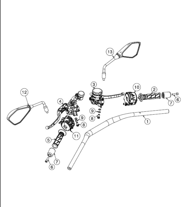
10.1 Handlebar
