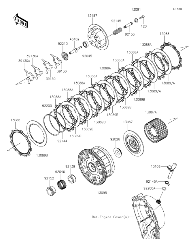
K9. Clutch
