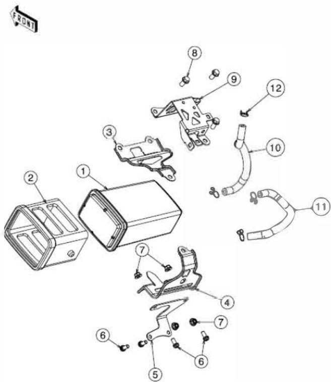
19 Canister
