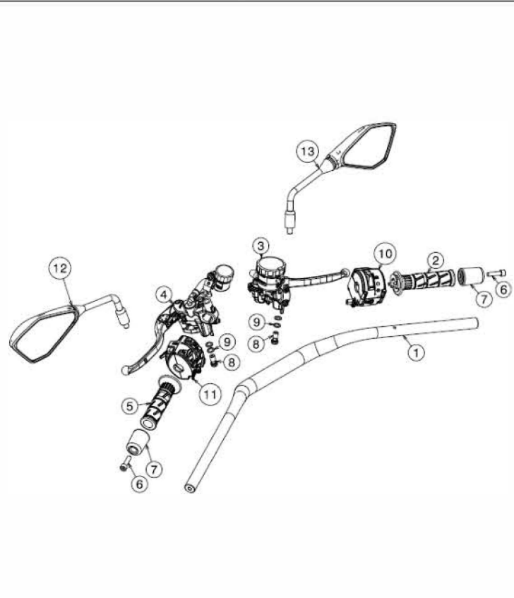
10.1 Handlebar
