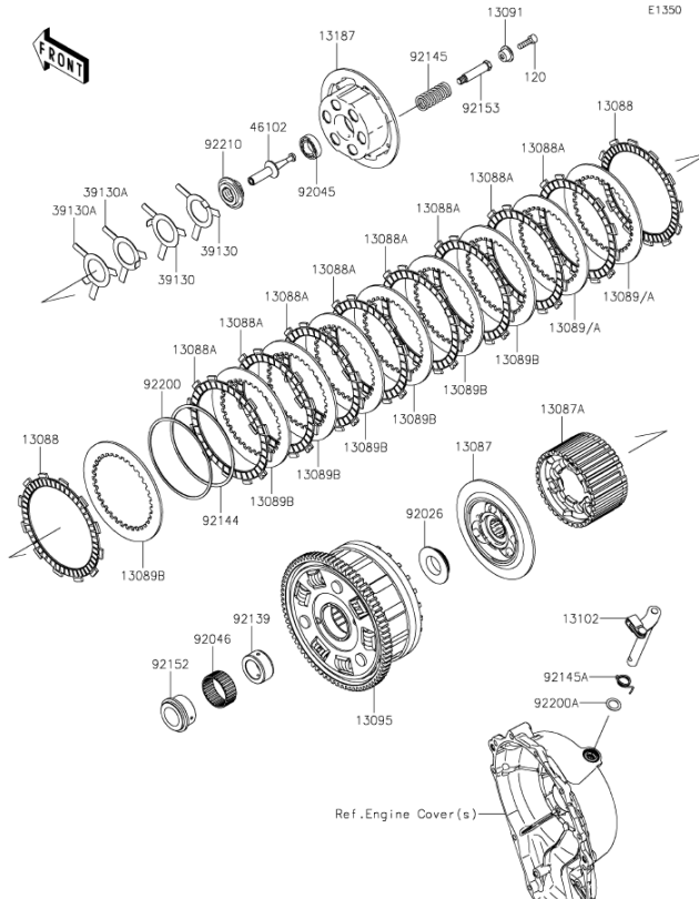
K9. Clutch
