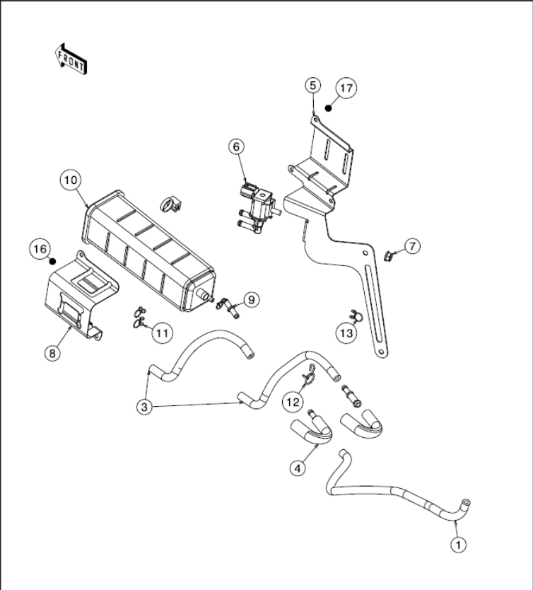
11. Canister
