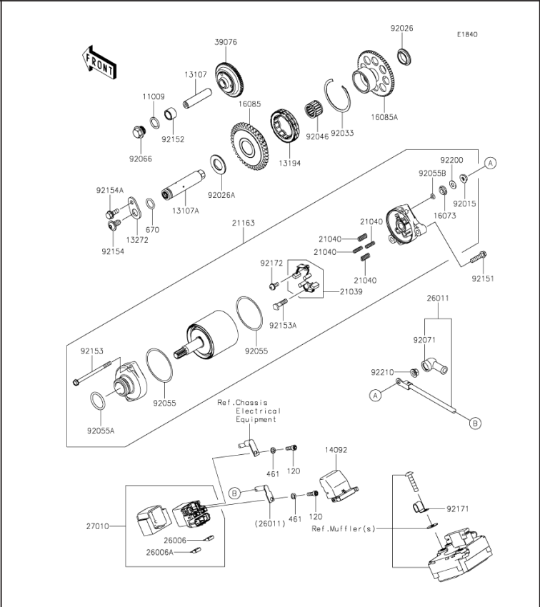
K24. Starter Motor
