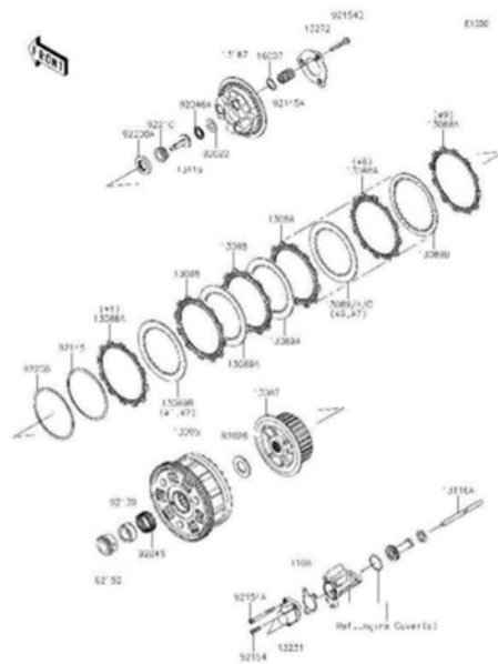
9 Clutch
