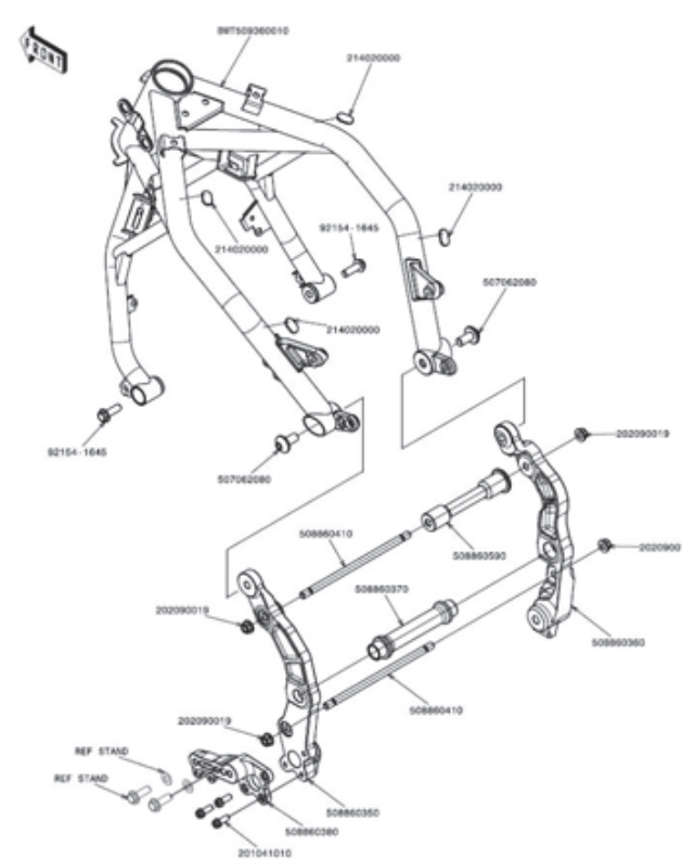
3.1 Frame
