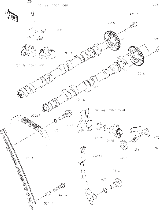
K7 Camshaft(s)/Tensioner
