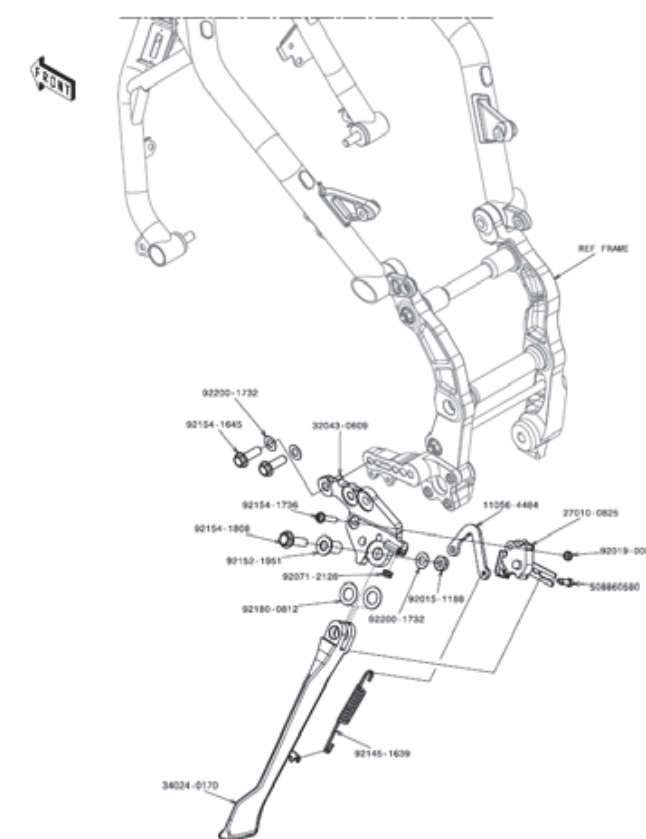
3.2 Frame (stand)
